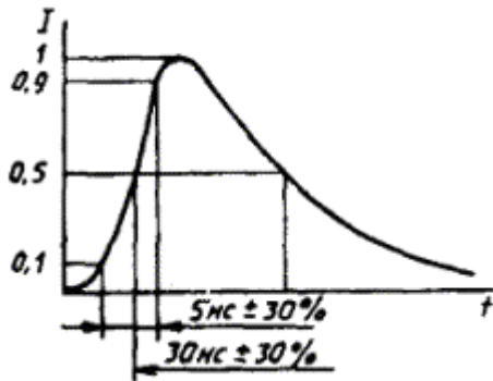
Рисунок Г.2 - Форма волны
