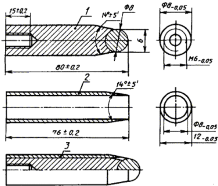
Рисунок Г.3 - Разрядный электрод
